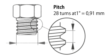
G 1/8" – outer-Ø = 9,6 mm
